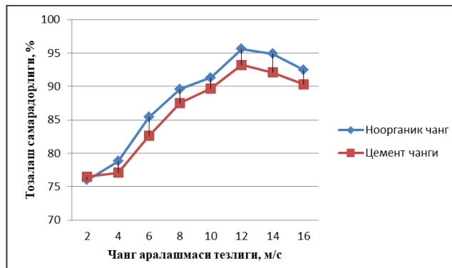
2-расм. Чанг аралашмалари оқими тезлигининг тозалаш самарадорлигига боғлиқлиги
