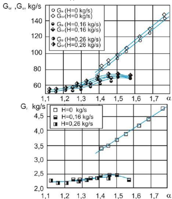
3-расм. Аралашманинг таркиби бўйича созлаш характеристикаси.
