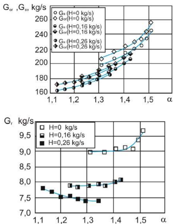
4-расм. Аралашманинг таркиби бўйича созлаш характеристикаси.
