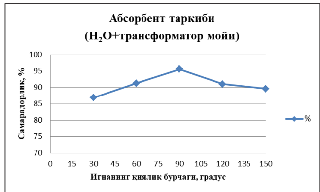
4-расм. Ускунага маҳкамланган игналарнинг қиялик бурчаги ҳамда абсорбент таркибининг (H 2 O+трансформатор мойи) тозалаш самарадорлигига боғлиқлиги
