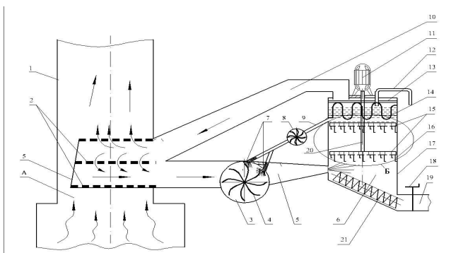
1-расм. Сув хўжалиги қурилиши корхонаси мўриконидан чиқаётган чиқинди газ ва чанг аралашмаларини тутиб қолувчи экспериментал ускунаси схемаси.
