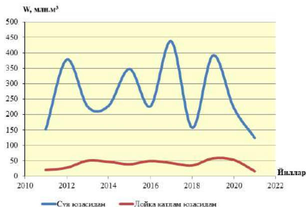
5-расм. Туямўйин сув омборлари мажмуасининг сув сатҳи ва лойқа қатлами юзасидан буғланишнинг кўп йиллик миқдори, млн м 3 .
