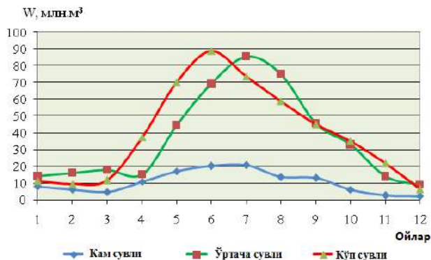
3-расм. Кам сувли, ўрта сувли ва кўп сувли йиллар учун Туямўйин сув омборлари мажмуаси сув юзасидан буғланиш ҳажмларининг йиллик тақсимланиши.
