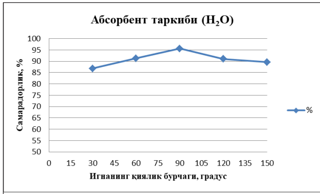
3-расм. Ускунага маҳкамланган игналарнинг қиялик бурчаги ҳамда абсорбент таркибининг (H 2 O) тозалаш самарадорлигига боғлиқлиги
