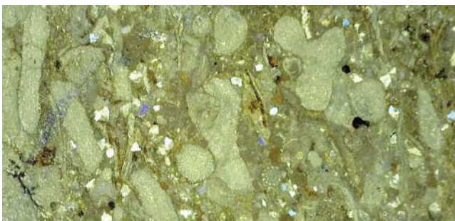
Рис.3. Шлиф ПТ-30/5. Многочисленные остатки водорослей (х-10) в отложениях верхнетахтатауской подсвиты P_2tt_3
